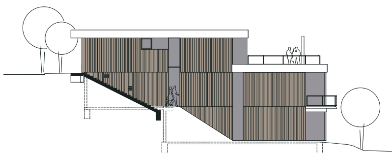
Ansicht Nord | Elevation North
