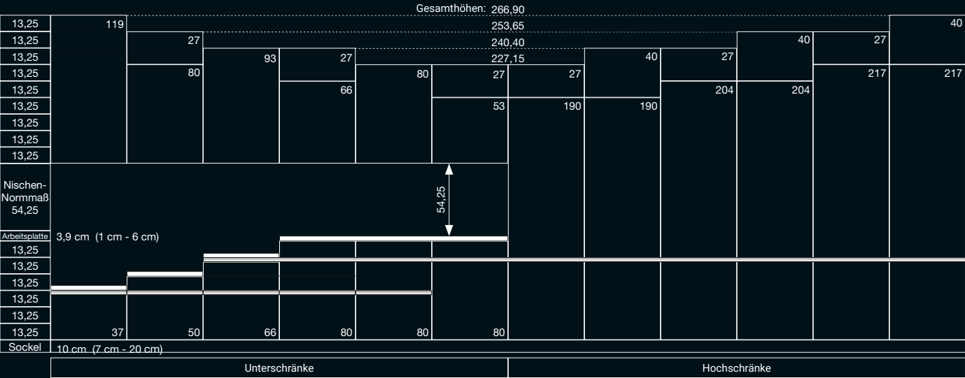
Oberschränke / Aufsatzschränke
